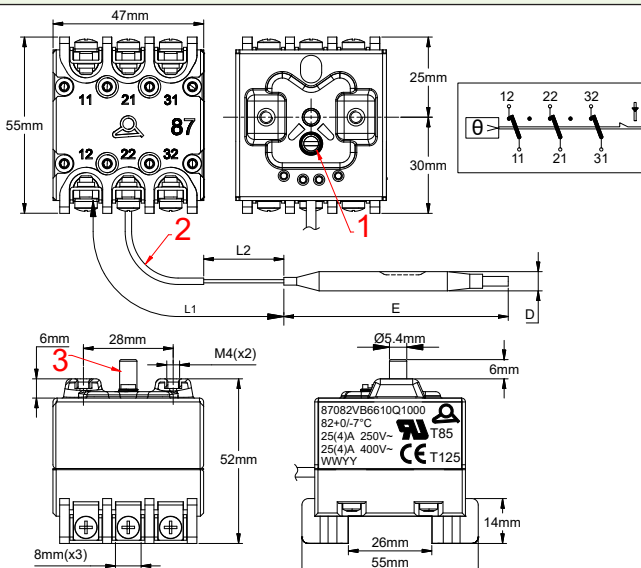
1. Siegelung; 2. Hülse; 3. Manueller Rückstellknopf
