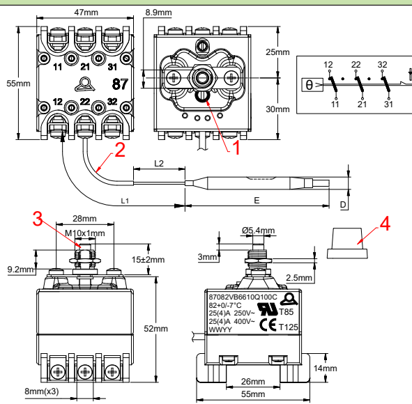
1. Siegelung; 2. Hülse; 3. Manueller Rückstellknopf; 4. Plastikkappe (schwarz)
